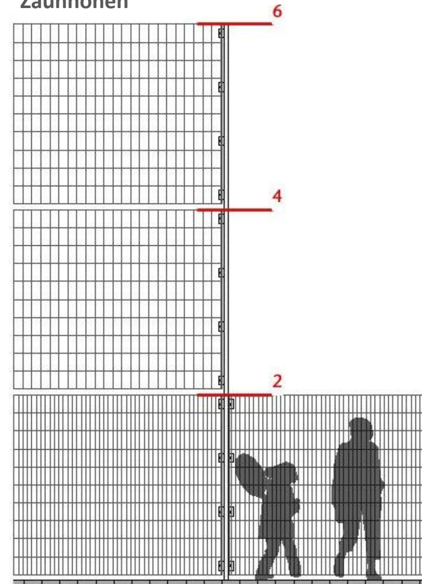
Zaunhöhen
